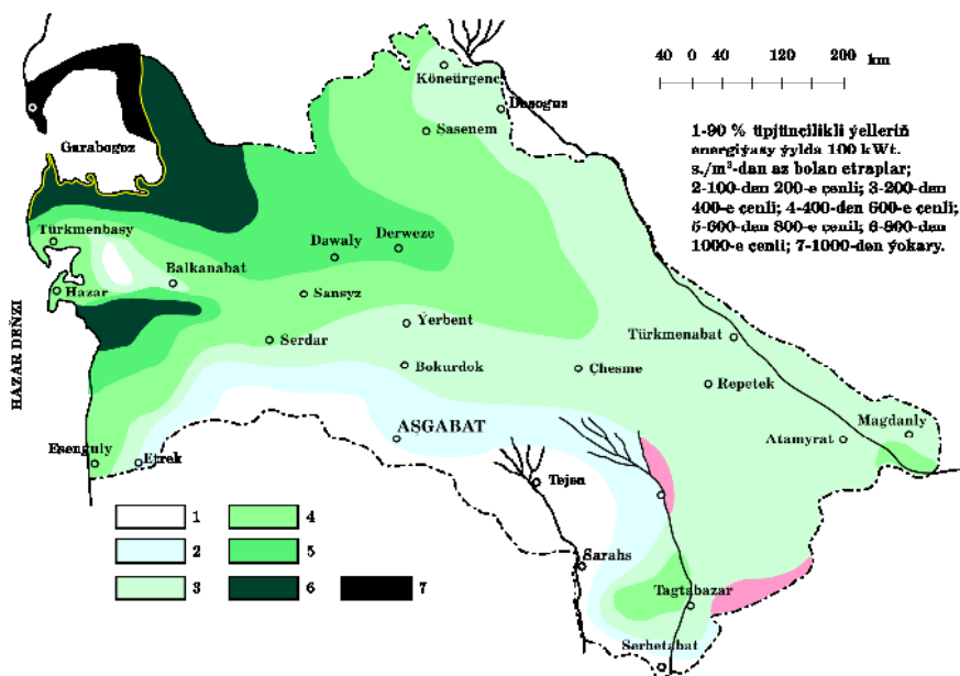
46-njy surat. Türkmenistanyň ýel energiýa baýlyklary
