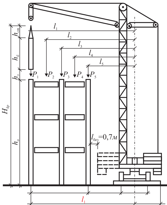
22-nji çyzgy. Başnyaly kranyň gerekli tehniki parametrlerini kesgitlemek üçin shema
