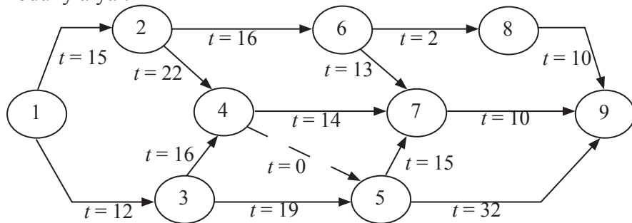
15-nji çyzgy. Set grafiginin parametrlerini tablisa usuly bilen hasaplamagyň shemasy
