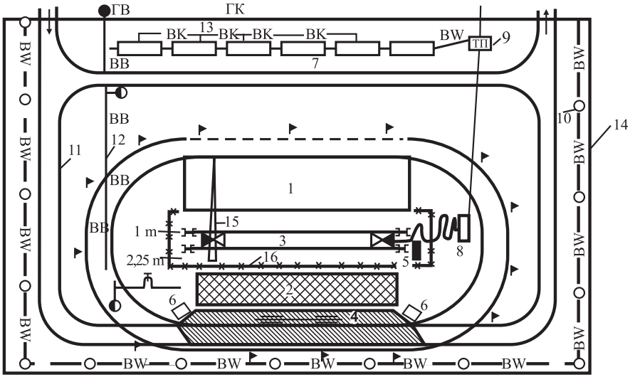
21-nji çyzgy. Başnyaly kran bilen gurnalýan köpgatly jaýyň baş gurluş meýilnamasy
