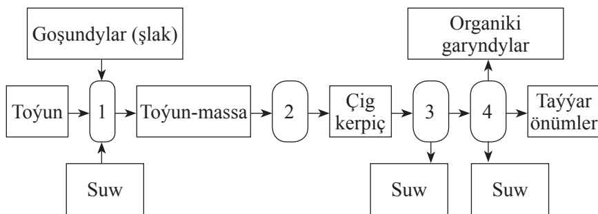
8.1-nji şekil. Şekil berlip keramiki kerpjiň we daşlaryň önümçiliginiň tehnologiýa hadysalarynyň zygiderligi: 1 – toýun massany taýýarlamak; 2 – önüme şekil bermek; 3 – guratmak; 4 – bişirmek
