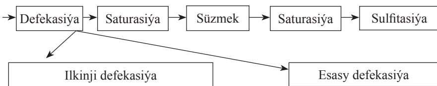
15.2-nji şekil. Diffuzion şiräni arassalamak tapgyrlary
