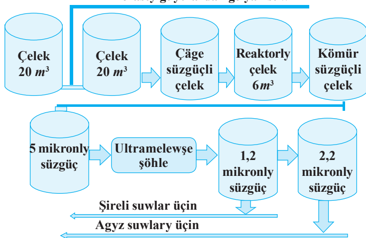
16.2-nji şekil. Suwuň arassalanylyş usuly
