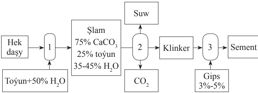
8.2-nji şekil. Portlandsementi çygly usul arkaly öndürilişiniň tehnologik hadysalarynyň çyzygysy
