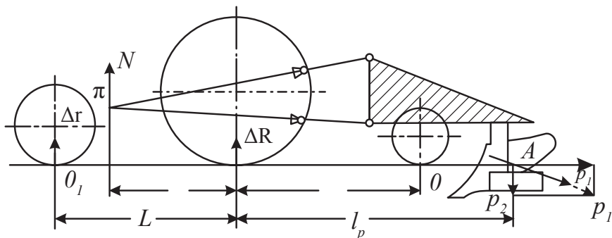
21-nji çyzygy. Azally traktoryň ilişme agramynyň kesgitlenilişi
