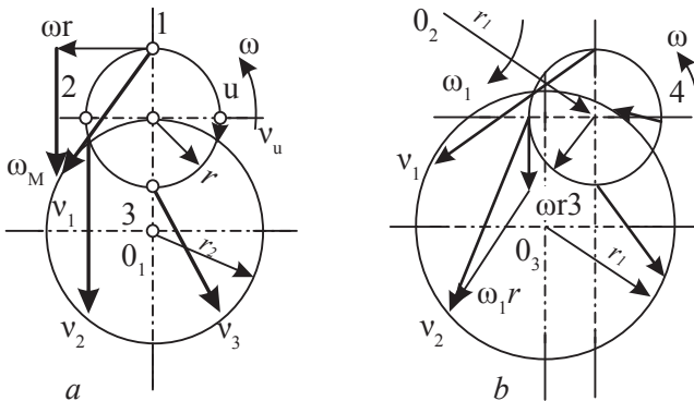
105-nji çyzgy. Dürli hereketde töwerek boýunça nokadyň absolyút tizligi
