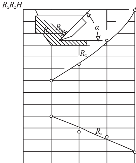
7-nji çyzgy. Düzüji güýçleriň burça ( \alpha ) görä üýtgeýşi
