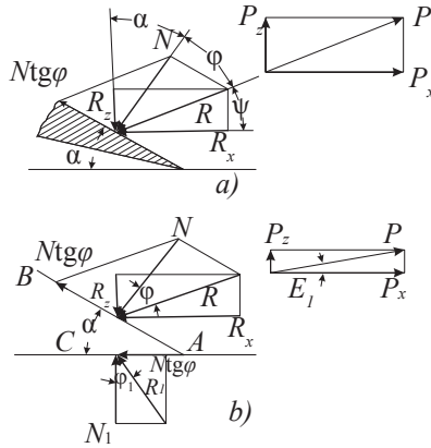
6-njy çyzgy. Pahna täsir edýän güýçler: a-ýönekeý pahna; b-iki taraply pahna
