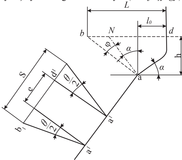
37-nji çyzgy. Ýumşadyjynyň iş enjamlarynyň ölçeglerini esaslandyrmak
