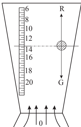
83-nji çyzygy. Konus görnüşli akabanyň iş hadysasy
