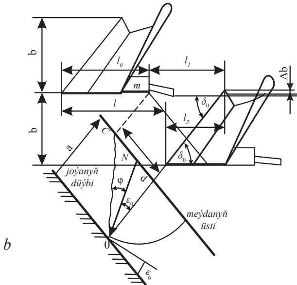
18-nji çyzygy. Azalyň iş gurallarynyň we tigrleriniň ýerleşdirilişi: a-ýerleşdirilişi; b-aralyklaryň kesgitenilişi
