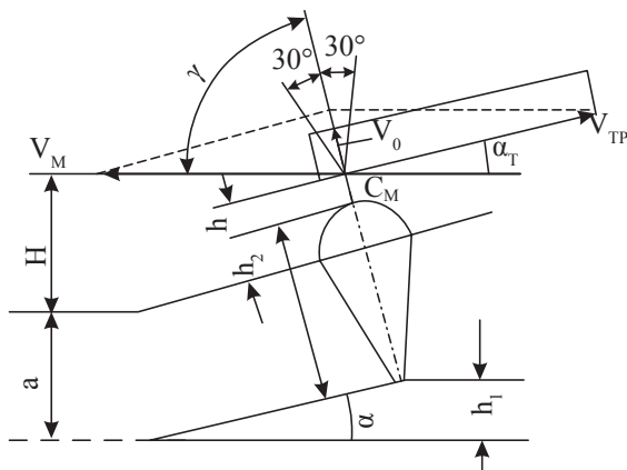
100-nji çyzgy. Kökleriň silkelenişiniň çyzgysy
