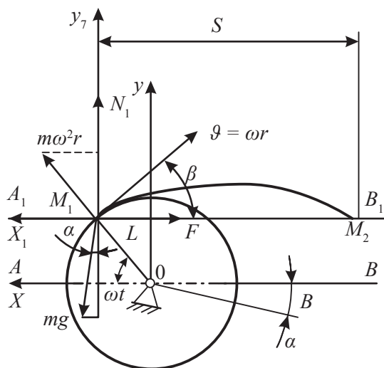
80-nji çyzygy. Klawişli saman silkeleýjiniň iş hadysasy
