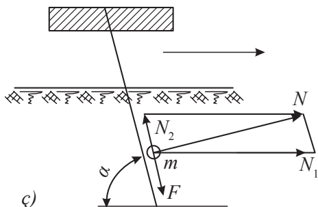
26-njy çyzgy. Dyrmygýň dişine täsir edýän güýçler we olaryň toprakdaky täsir güýji
