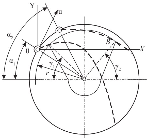
95-nji çyzgy. Saýlaýjynyň (triyer) kabul edýän bölejiginiň ýerleşşi
