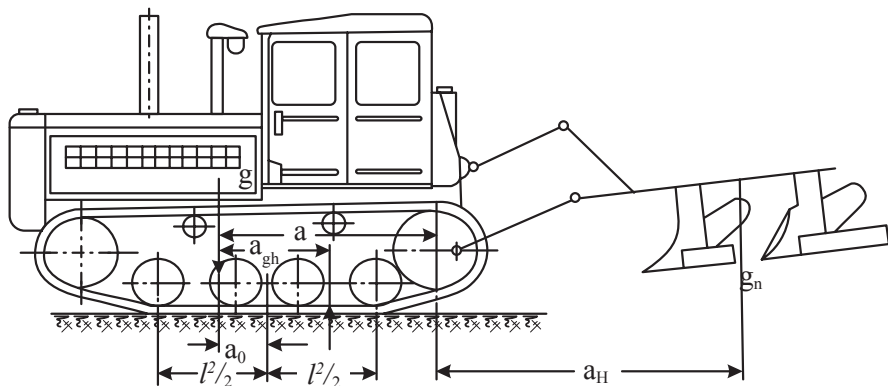
24-nji çyzgy. Zynjyrlý traktora dakylan asma azalyň uzaboý meýdança boýunça durnuklylygynyň hasaplamlary
