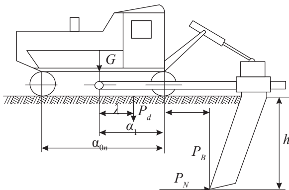
122-nji çyzyg. Asma topragy ýumşadyja we kesijä täsir edýän güýçler
