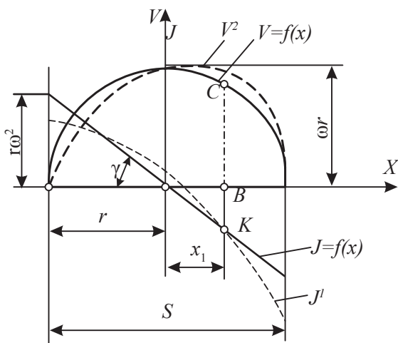
58-nji çyzgy. Pyçagyň hereketine baglylykda tizliginiň we tizlenmäniň üýtgeýişi
