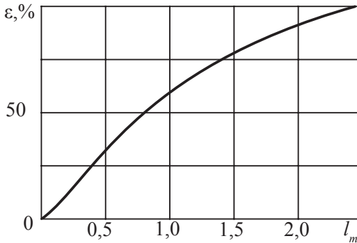
88-nji çyzgy. Dykzlygyň görkezijisiniň elegiň uzynlygyna görä üýtgeýşi
