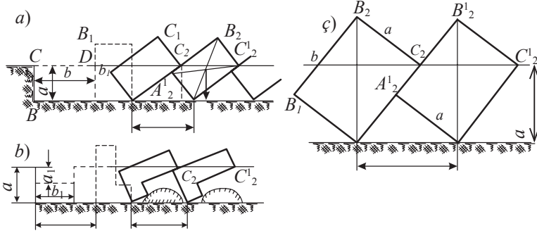
13-nji çyzygy. Kündäniň täsiri bilen toprak gatlagynyň aýlanyşy: a-azalçasyz; b-gatlagyň eýeleýän ýagdaýy; ç-azalçaly
