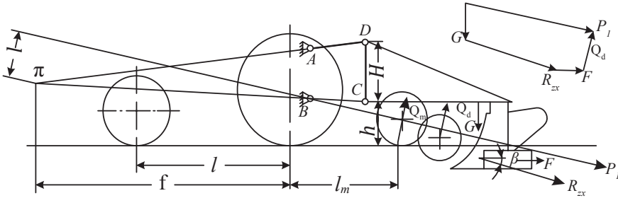
20-nji çyzygy. Azalyň asma ulgamynyň birikdiriji nokatларыnyň ýerleşşi
