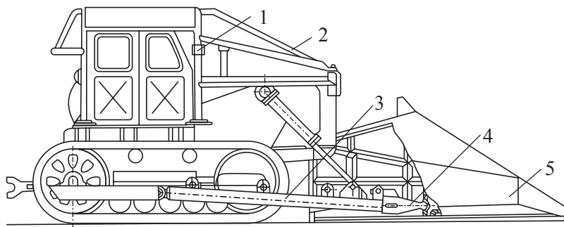
118-nji çyzgy. Gyrymsy agaçlary kesýän maşynyň gurluşy
