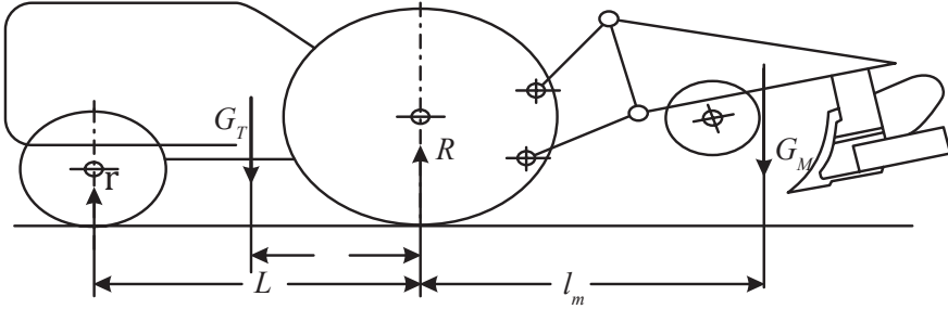
23-nji çyzgy. Tigirli traktora dakylan asma azalyň uzaboýy meýdança boýunça durnuklylygynyň hasaplamalary
