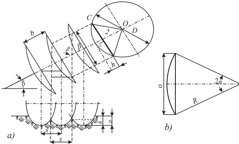
29-njy çyzgy. Tegelek iş enjamly dyrmyklaryň hasaplamalarynyň çyzgysy: a – enjamlaryň dyrmygyň süňnünde ýerleşşi; b – güberçek tegelek
