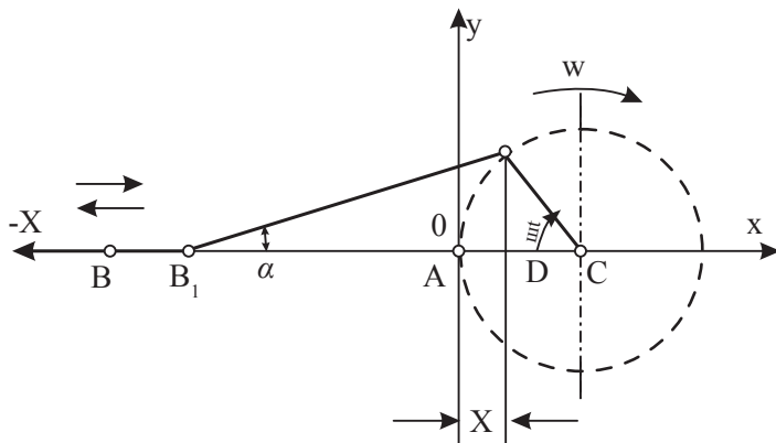
57-nji çyzgy. Pyçagyň süýşýän aralygyny kesgitlemek
