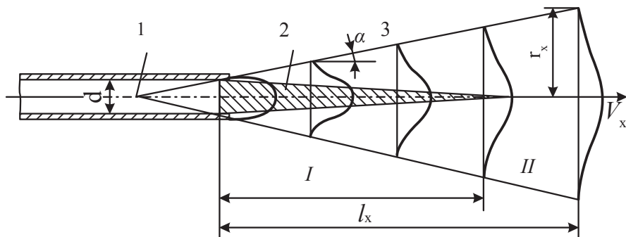
47-nji çyzgy. Pürkujiden çykýan suwuklygyň hereketi
