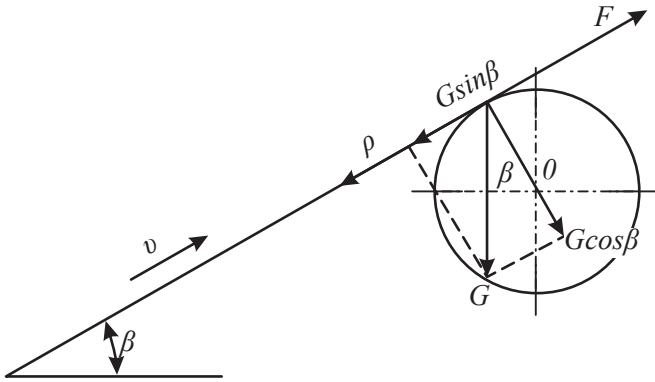
70-nji çyzgy. Transportýoryň (süýşürijiniň) ýapgytlyk burçuny kesgitlemek
