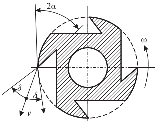
104-nji çyzygy. Şpindeliň dişleriniň ýokarsynyň tizliginiň ugry
