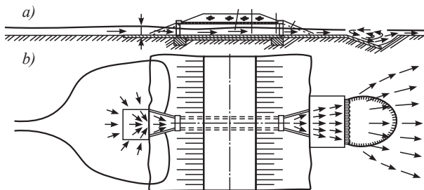
22-nji surat. Akymyň suw geçiriji desgadan geçişiniň çyzygysy: a – akabanyň uzynlygyna profili; b – meýilnamasy.
