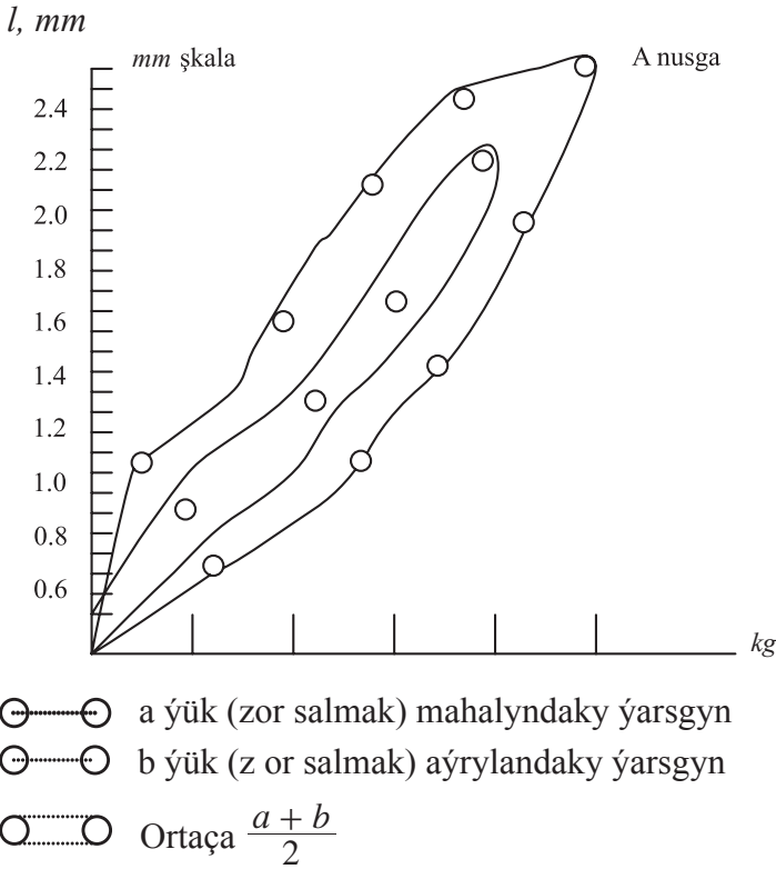
5-nji surat. Materialyň süýnüşiňiň (uzaýşynyň) we ýüküniň (zor salmagyň) aýrylyşynyň diagrammasy
