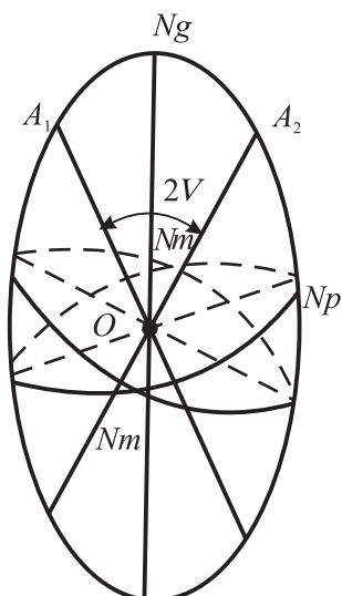
9-njy surat. Aşaky kategoriýa singoniýalarynyň kristallarynyň optik indikatrişasy
