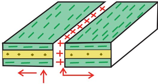
45-nji surat. Dik we ýapgyt daýkalaryň, ýagny döwürme jaýrylmalaryň görnüşleri
