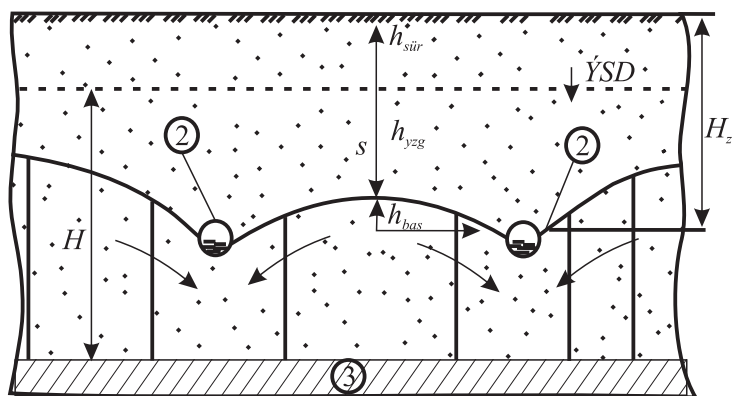
39-nji surat. Suwarymly ýerlerde suwuň derejesiniň zeýkeş turbalary arkaly pese düşürilişi:
