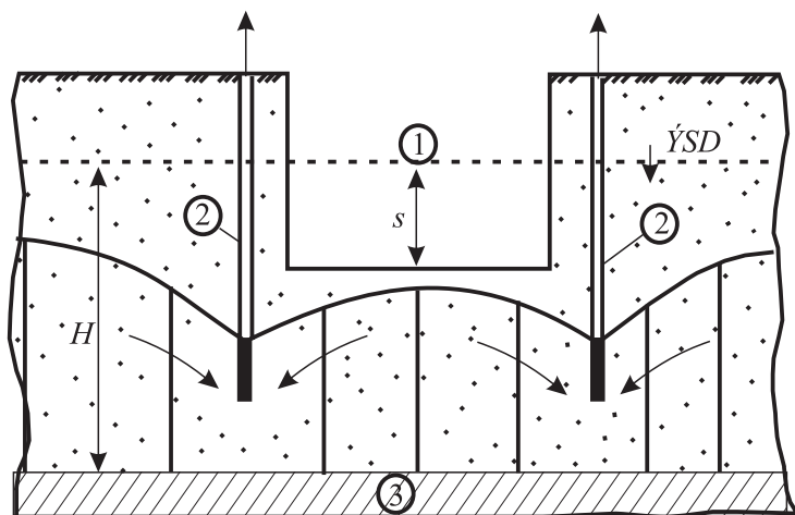
38-nji surat. Gurluşyk hendegindäki suwuň derejesiniň zeýkeş guýulary arkaly pese düşürilişi:
