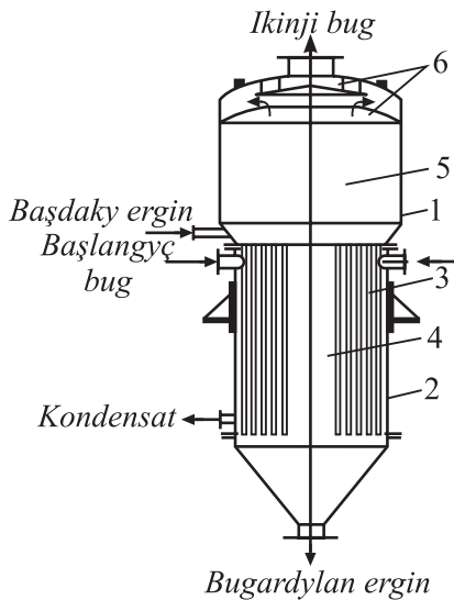
10.7-nji surat. Içi gyzdyryjy kameraly we merkezi aýlanyşyk turbajykly bugartma aparaty:
