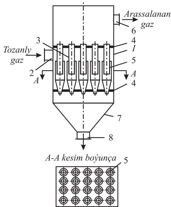
6.4-nji surat. Batareýli siklon:
