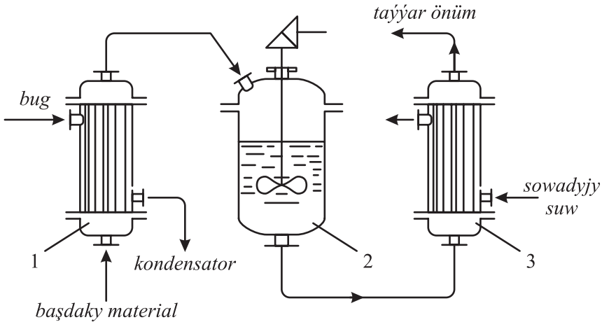
1.3-nji surat. Üznüksiz proses boýunça işleýän desganyň takmynan (prinsipial) shemasy:
