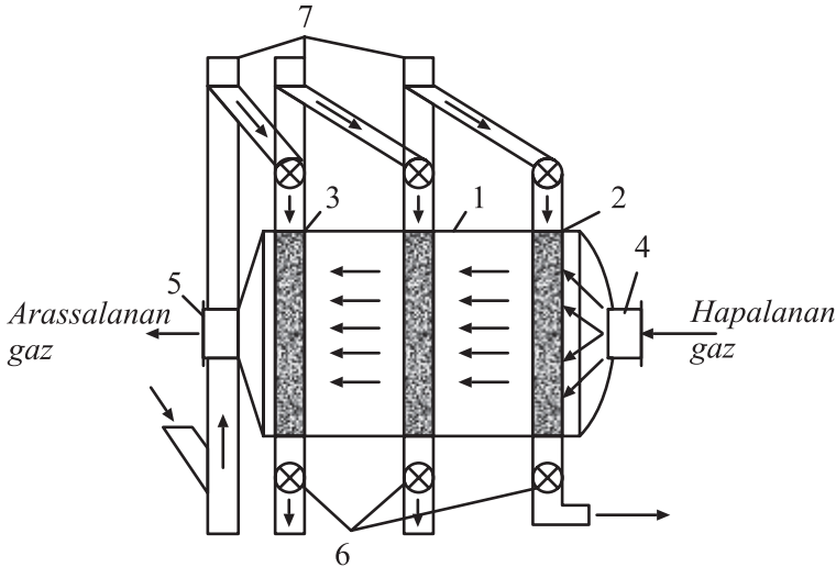
6.7-nji surat. Hereketlenýän däne görnüşli süzüji material gatlagy bolan üznuksiz işleýän filtr:
