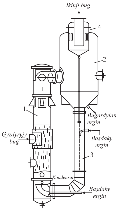
10.10-njy surat. Çykarylan gyzdyryjy kameraly bugardyjy aparat: 1 – gyzdyryjy kamera; 2 – separator; 3 – gyzdyrylmaýan aýlanyşyk turbasy; 4 – pürkülmäni tutujy
