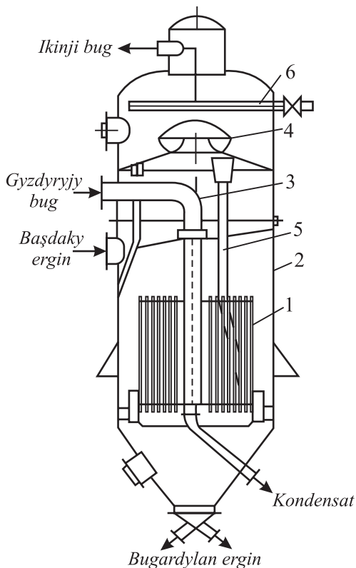
10.8-nji surat. Asma gyzdyryjy kameraly bugardyjy aparat:
