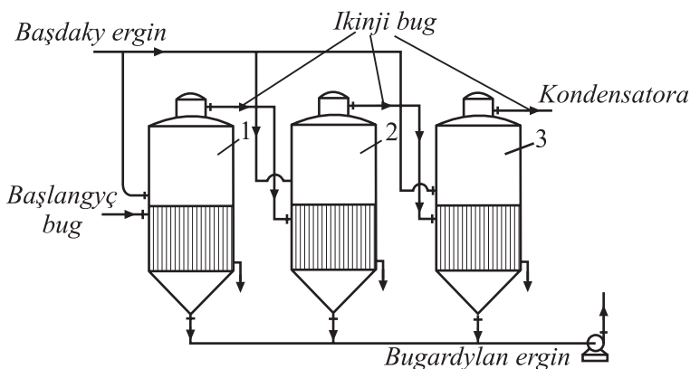
10.4-nji surat. Korpuslary parallel ýmitlendirilýän (kabal edýän) köp korpusly bugartma desgasy (1-3)
