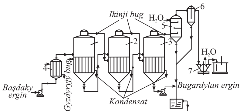
10.2-nji surat. Köp korpusly ugrundaş akymly wakuum-bugartma desgasy: 1-3 – bugartma aparatlarynyň korpuslary; 4 – başdaky ergini gyzdyrmak üçin ýylylyk çalşyjy apparat; 5 – barometriki kondensator; 6 – tutujy aparaty; 7 – wakuum-nasos
