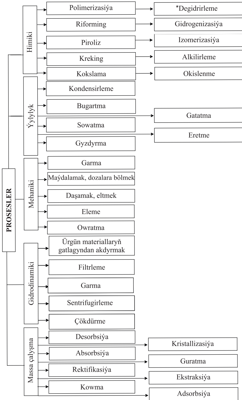
1.1-nji surat. Himiýa tehnologiýasynyň esasy prosesleriniň toparlara bölünmesiniň shemasy
