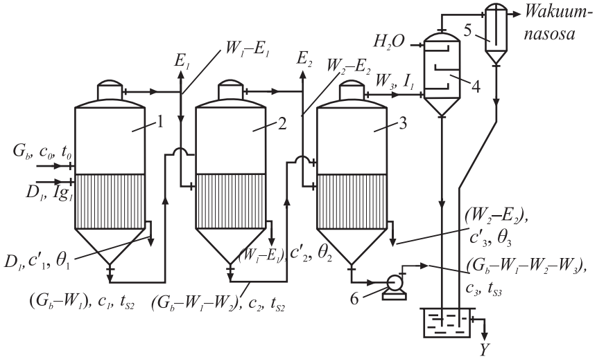
10.5-nji surat. Köp korpusly bugartma desgasynyň ýylylyk balansyny düzmek üçin tehnologiki çyzgy:
