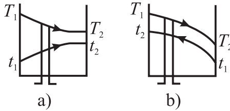
8.13-nji surat. Ýylylyk äkidijileriň temperaturalarynyň üýtgeýişi: a – göni akym; b – garşylykly akym
