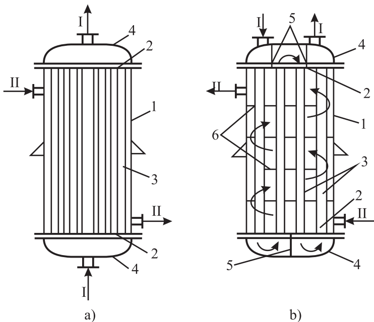
9.3-nji surat. Gabyk turbaly bir ýörişli (a) we köp ýörişli (b) ýylylyk çalşyjy apparatlar:
