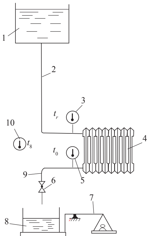
4-nji surat. Gyzdyryjy enjamyň ýylylyk alyp-beriş koeffisiýentini kesgitlemek üçin tejribe desgasynyň çyzzgysy
