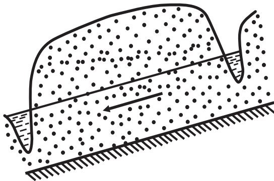
58-nji surat. Ýapgyt suwabent düşekde teýgum suwlarynyň deňölçeqli hereketi
