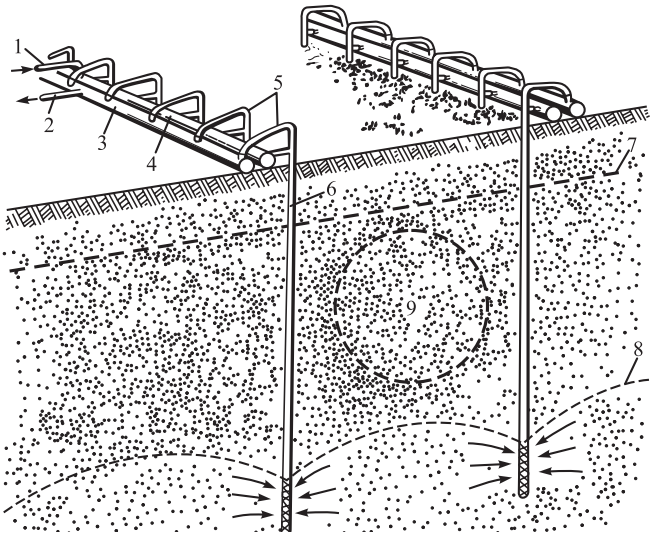
102-nji surat. Ežektorly iňňepisint süzgüç gurnamasynyň işleýiş shemasy:
