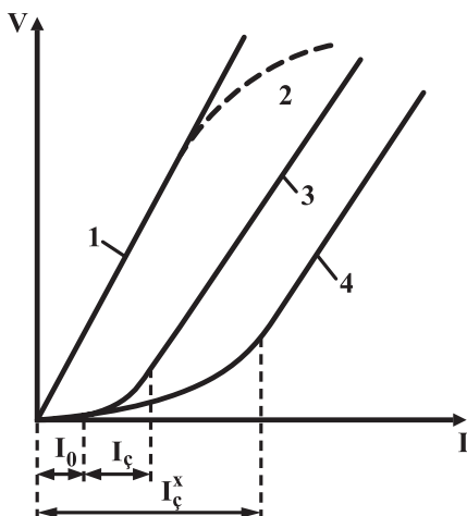
56-njy surat. Süzülmäniň esasy kanunlarynyň çyzgy şekili:
