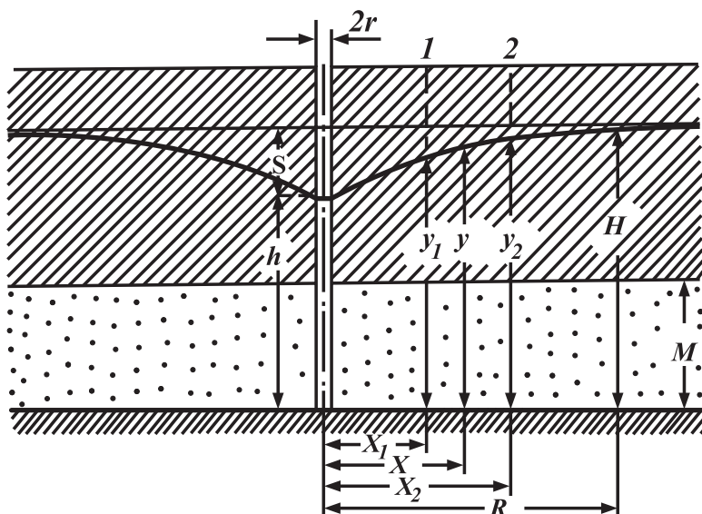
67-nji surat. Dyňzawly kämil guýa syzylp geljek suwuň hasaby üçin kömekçi çyzgy:
