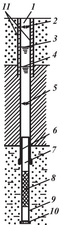
74-nji surat. Hidrogeologik skwažinanyň konstruksiýasynyň esasy elementleri:
