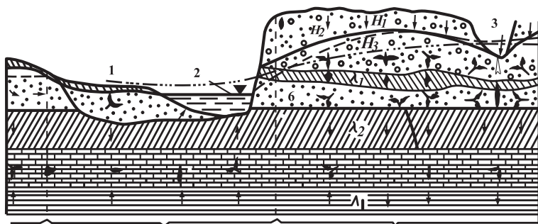
63-nji surat. Derýaaralyk ýaýlasynyda teýgum suwlarynyň hereketiniň çyzygysy (A.N.Mätiýew boýunça):
