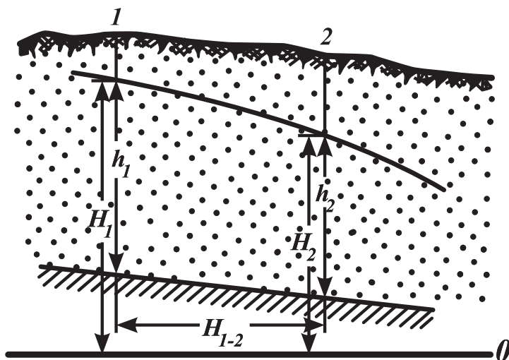
61-nji surat. Ýapgyt suwabentli teýgum suwларыnyň akymynyň hasaby üçin kömekeçi çyzgy
