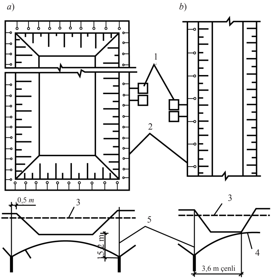
8-nji surat. Bir ýarusly iňňesüzgüji bilen guratmaklygyň shemasy
