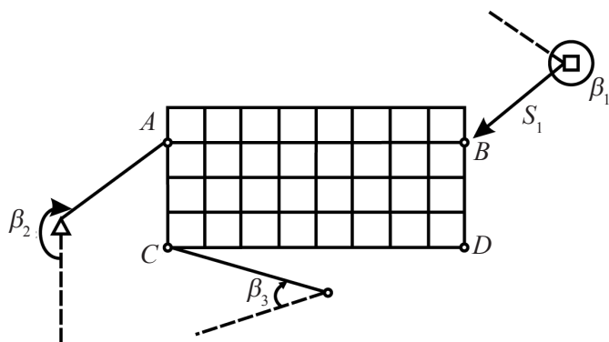
2-nji surat. Meýdana gurluşyk setkasyny çykarmaklygynyň shemasy
