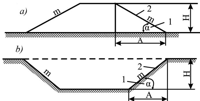
16-njy surat. Gazylan we üýşürilen topragyň ýapgydynyň elementleri 1 – ýapgyt burç, 2 – ýapgyt
