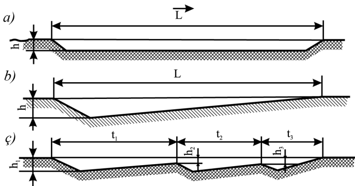
31-nji surat. Skreperiň topragy dürli görnüşde kesilişine görä zaboýyň ugruna kesiliş shemasy.
