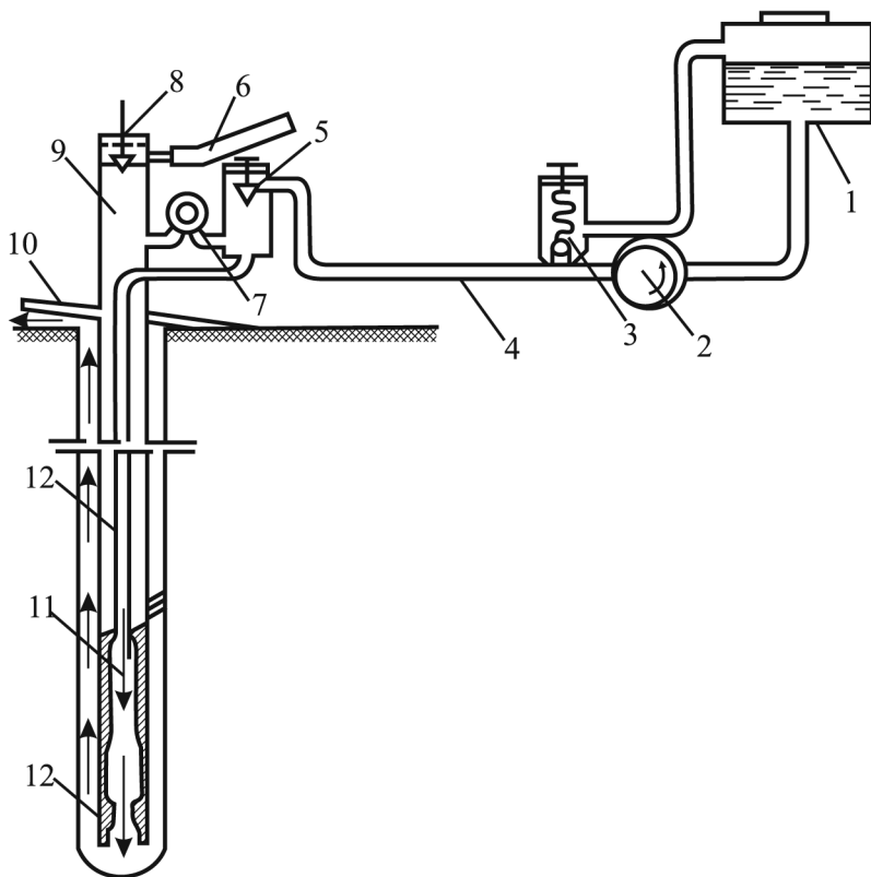
49-njy surat. RTB-B1 görnüşi we termoburawyň shemasy.
