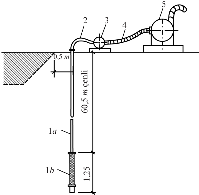
5-nji surat. Ýeňil inñesüzgüç gurmasy (YE.I.G-LIU)
