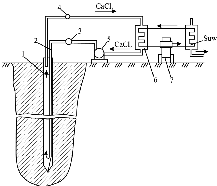
22-nji surat. Topragy berkitmekligiň gurmasynyň shemasy.
