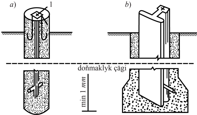
3-nji surat. Hemişelik toprak bellikleri
