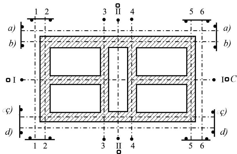
17-nji surat. Jaýlaryň oklaryny oturgyçlaryň kömegi arkaly berkitmek bilen jaýlary bölmeklik
