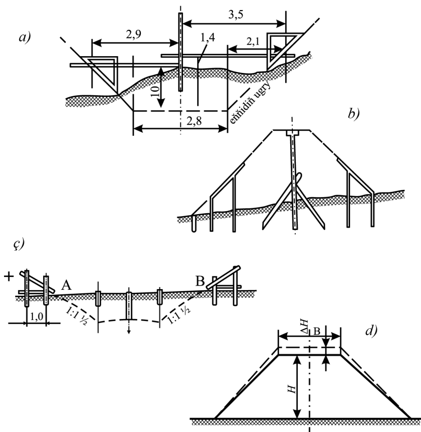
19-njy surat. Uly uzakly gazymalary we üşürimleri bellemekligiň shemalary.
