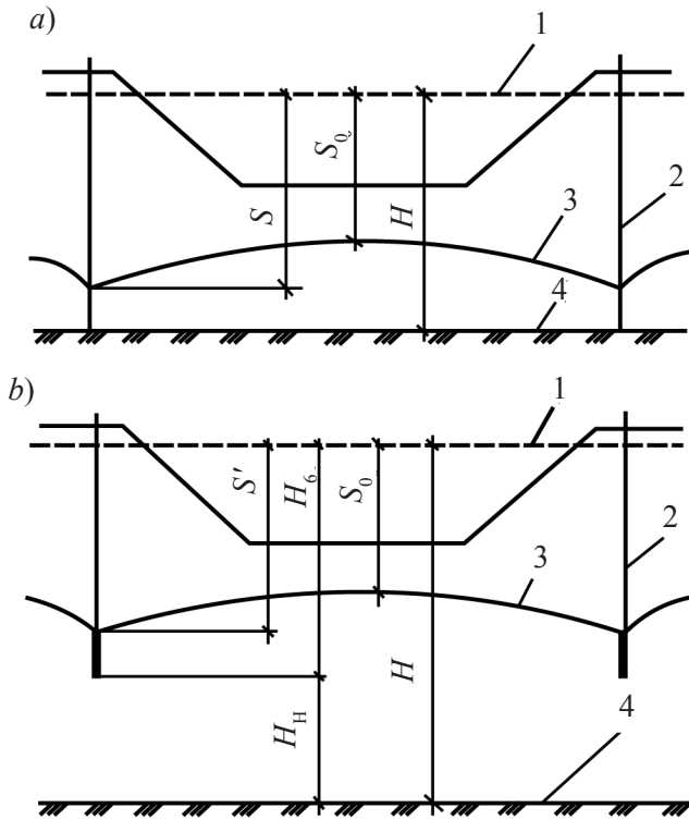
10-njy surat. Gaptaldan goşulma suw akymynyň garaşma mukdaryny kesgitlemegiň gurlalaryň shemasy
