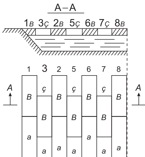
32-nji surat. Topragy şahmat-grebençatly kesmekligiň shemasy (zolaglaryň işleniş tertibini sanlar görkezýär; harp bolsa bir aýratyn zolagyň yzygiderli işlenişini görkezýär)
