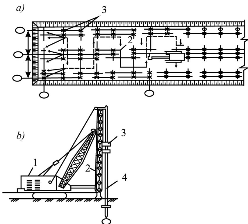
68-nji surat. Kran-ekskawatoryň bazasynda gazykuruujy gurulma bilen gazyklary kakmaklygyň shemasy
