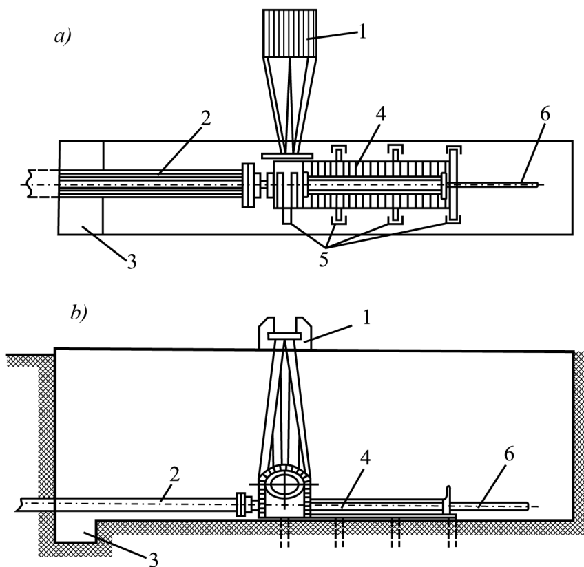
46-njy surat. Moseýrastygurluşygynyň gorizontel burawlamak üçin gurma shemasy.
