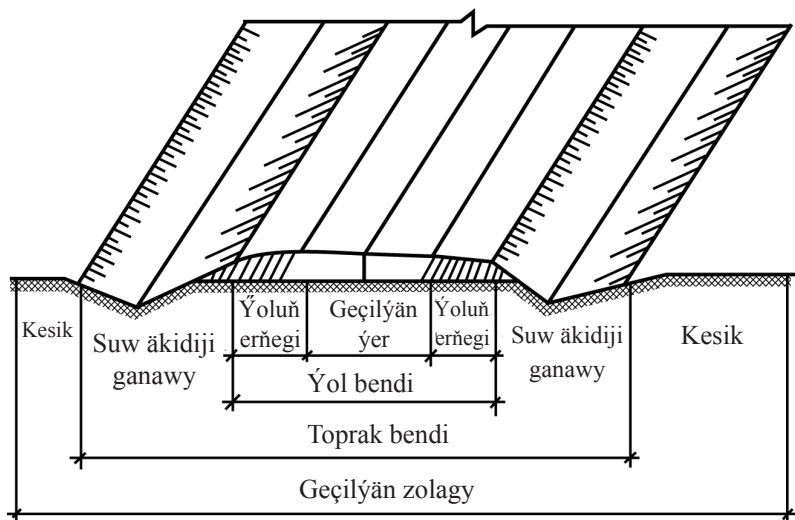
11-nji surat. Awtomobil ýolunyň kese profiliniň elementleri
