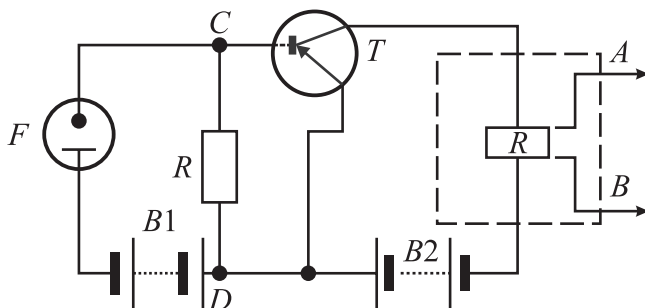
5.14-nji surat. Fotoelektriki dolandyrjy gurluş
