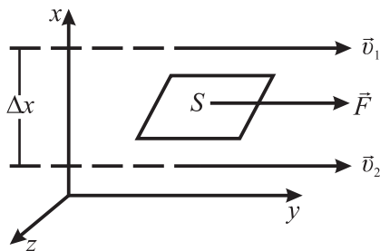
3.4-nji surat. Suwuklyklarda içki sürtülme güýji
