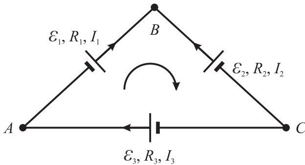
4.18-nji surat. Ýapyk elektrik zynjyry (kontur)
