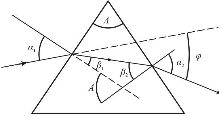
5.9-njy surat. Üçgranly prizmada ýagtylygyň döwlişi
