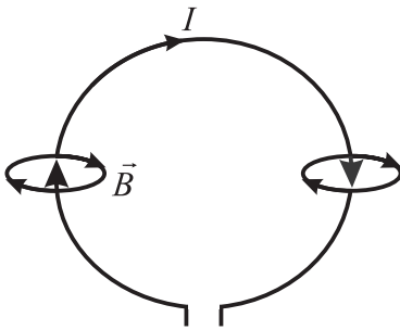
4.22-nji surat. Halka görnüşli toguň magnet induksiýasy
