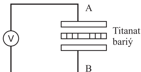
2.7-nji surat. Ultrases generatorynyň gurluşy
