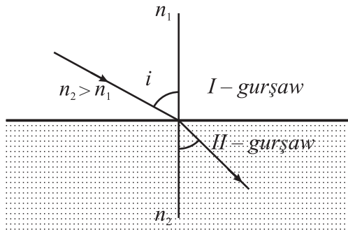
5.4-nji surat. Ýagtylygyň döwülme kanuny
