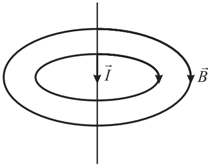
4.21-nji surat. Göni toguň magnet induksiýasy
