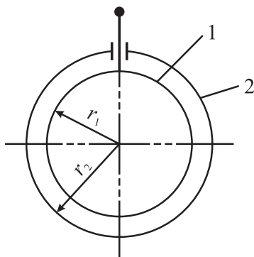
4.12-nji surat. Sferik kondensatoryň sygymynyň kesgittenilişi
