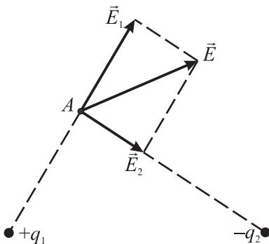
4.4-nji surat. Elektrik meýdanlarynyň üstüne goýma düzgüni
