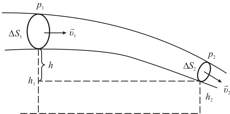
1.11-nji surat. Bernulliniň deňlemesiniň kesgitlenilşi
