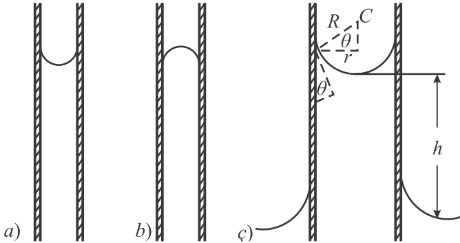
3.9-njy surat. Inçe turbalarda suwuklygyň üstüniň egrelişi
